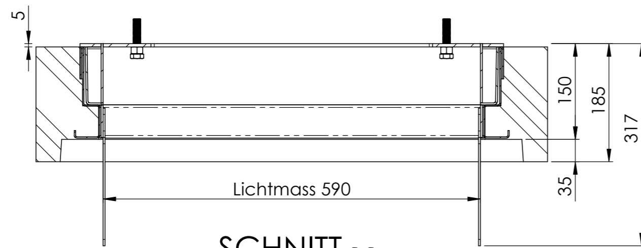
SCHNITT B-B
